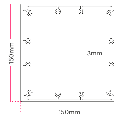
6 Column 150X150
