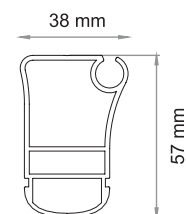
④ vidus profils средний профиль narrow counterweight
