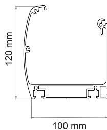
⑥ parapeta priekšējais profils профиль парапета gutter parapet
