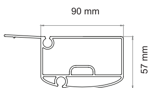
② apakšējais profils нижний профиль broad counterweight, bottom
