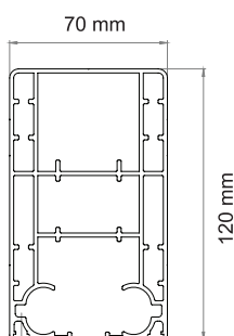
① sija балка guide
